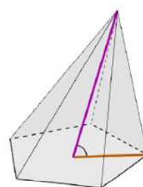
斜角錐
