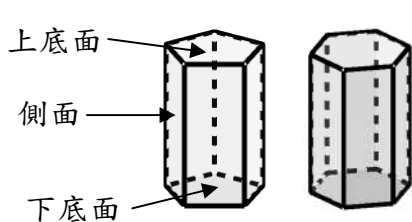
直角柱
