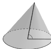
斜圓錐
