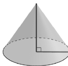
直圓錐
