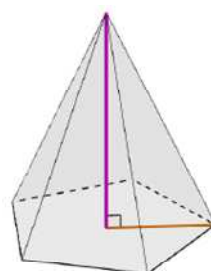
正角錐
